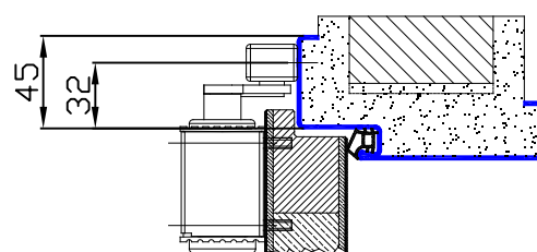
Sonderausführung Mit Spiegelverbreiterung auf der Falzseite
