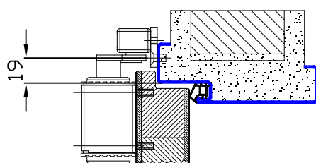
Standardausführung Vorgerichtet für bauseitige Scharnierplatte
