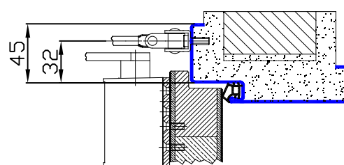
Sonderausführung Mit Spiegelverbreiterung auf der Falzseite
