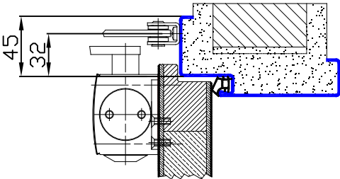
Sonderausführung Mit Spiegelverbreiterung auf der Falzseite
