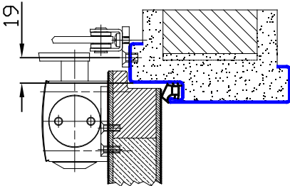
Standardausführung Vorgerichtet für bauseitige Scharnierplatte
