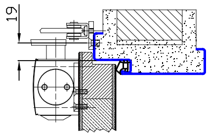
Standardausführung Vorgerichtet für bauseitige Scharnierplatte
