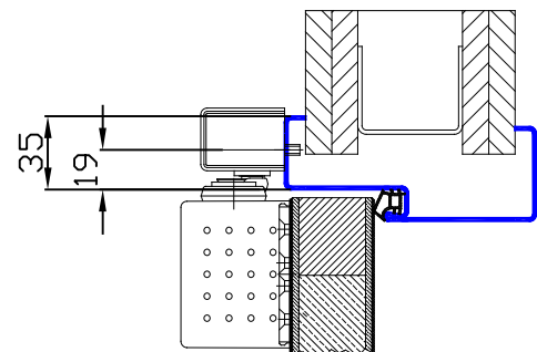
Standardausführung Mit Spiegelverbreiterung auf der Falzseite
