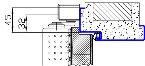
Standardausführung Mit Spiegelverbreiterung auf der Falzseite
