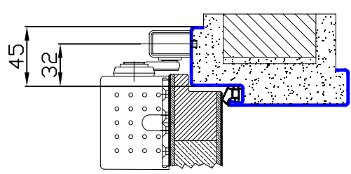
Sonderausführung Mit Spiegelverbreiterung auf der Falzseite
