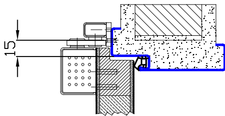
Standardausführung Vorgerichtet für bauseitige Scharnierplatte
