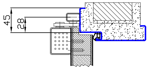
Sonderausführung Mit Spiegelverbreiterung auf der Falzseite
