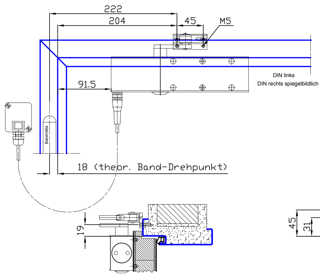
Standardausführung Vorgerichtet für bauseitige Scharnierplatte
