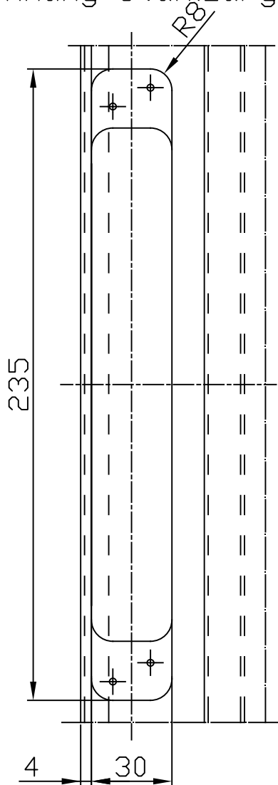
Ausnehmung Stahlzarge
