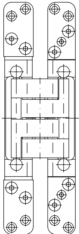
Ausnehmung Stahlzarge
