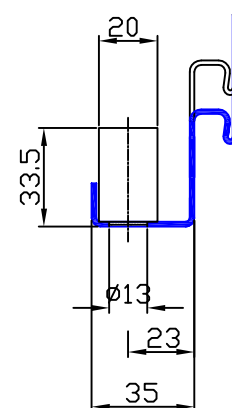
Anuba Anschweißklotz AKL (653)
